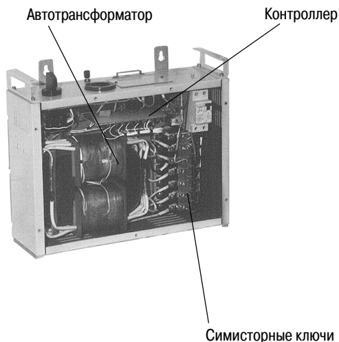
Рис. 8. Устройство стабилизатора
