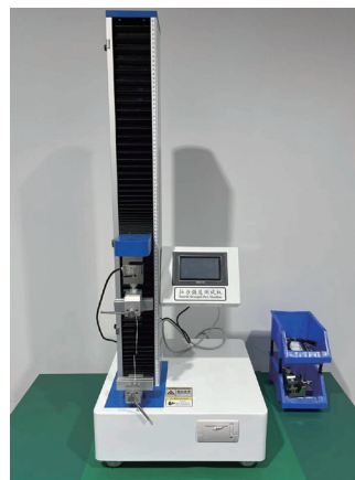
Tensile Strength Tester
